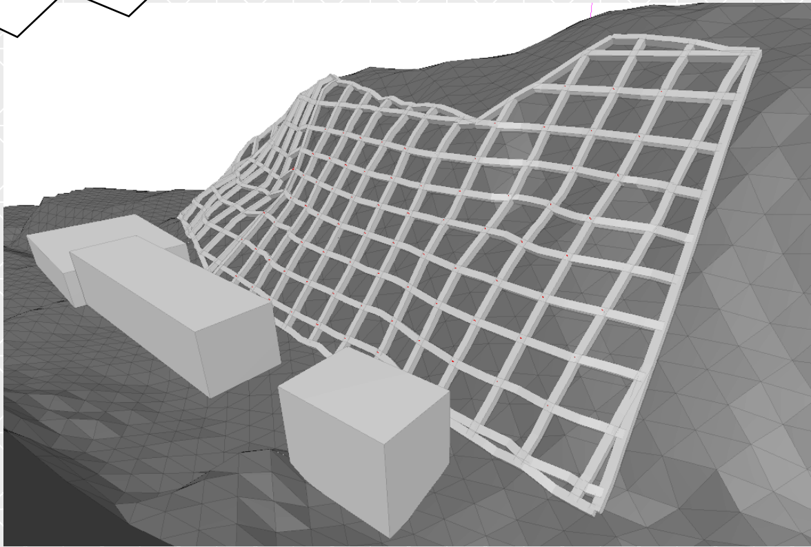
3次元CADで法枠を配置
