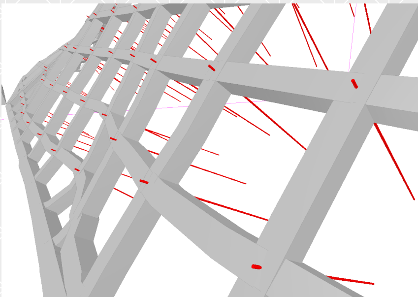
アンカー（鉄筋挿入工）を配置
